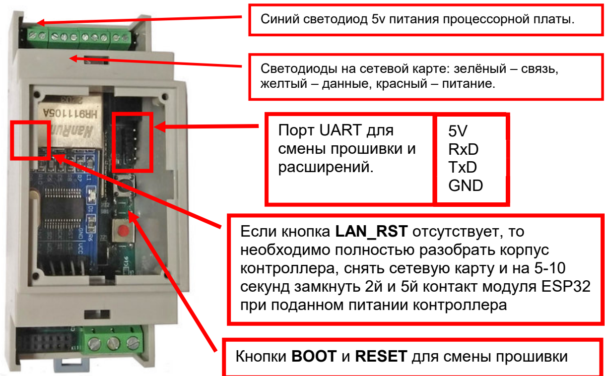
Рисунок 5 – расположение кнопок и порта UART на плате контроллера.
