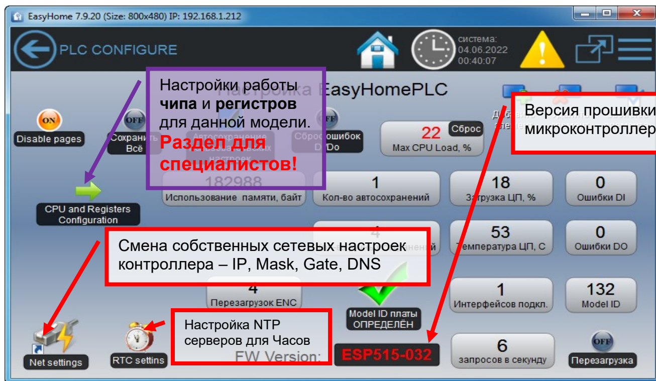
Рисунок 9 – главная страница конфигурации контроллера
