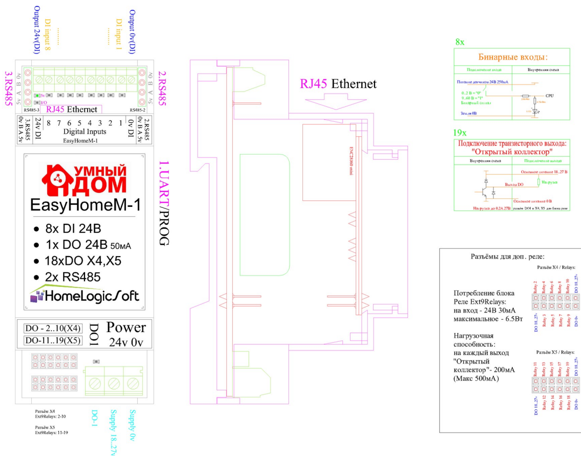
Рисунок 1 – клеммы контроллера
