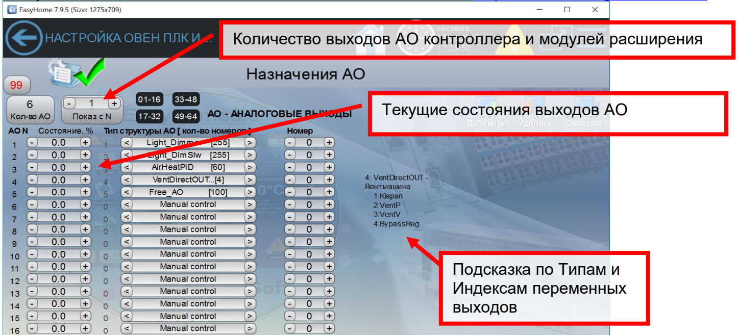
Рисунок 14 – настройка аналоговых выходов контроллера
