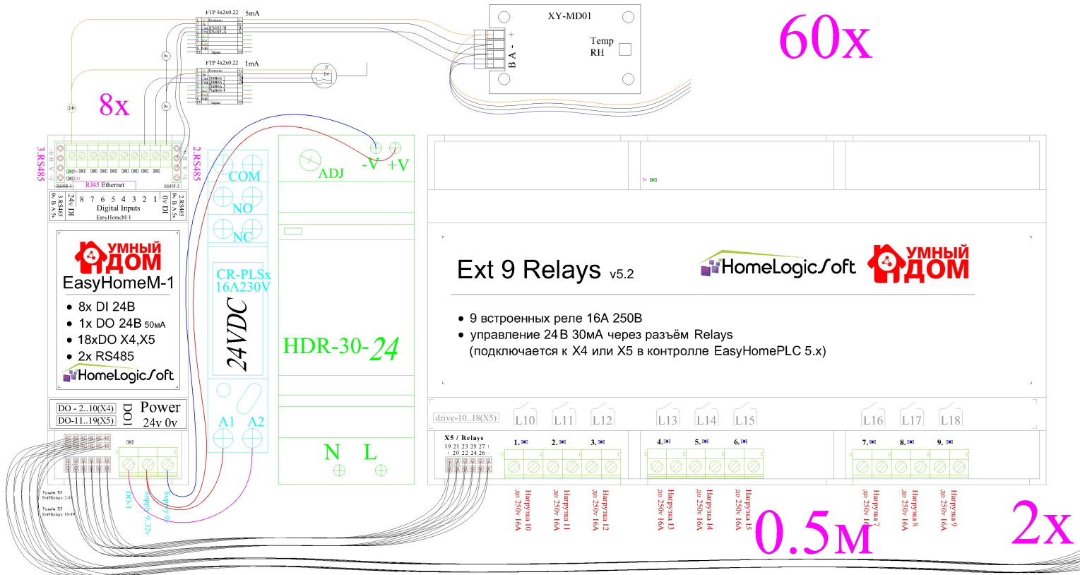
Рисунок 2 – типовые подключения контроллера
